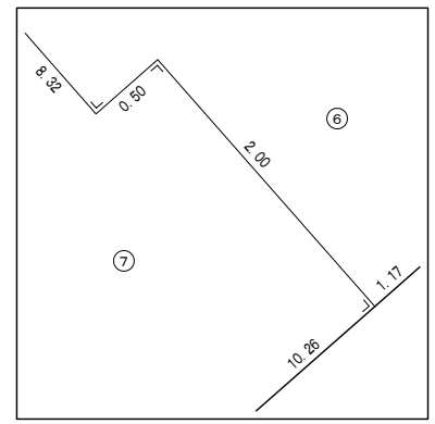
拡大図 1/50
