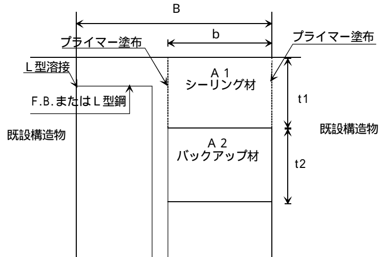
目地幅が広い場合の改良（参考図）
