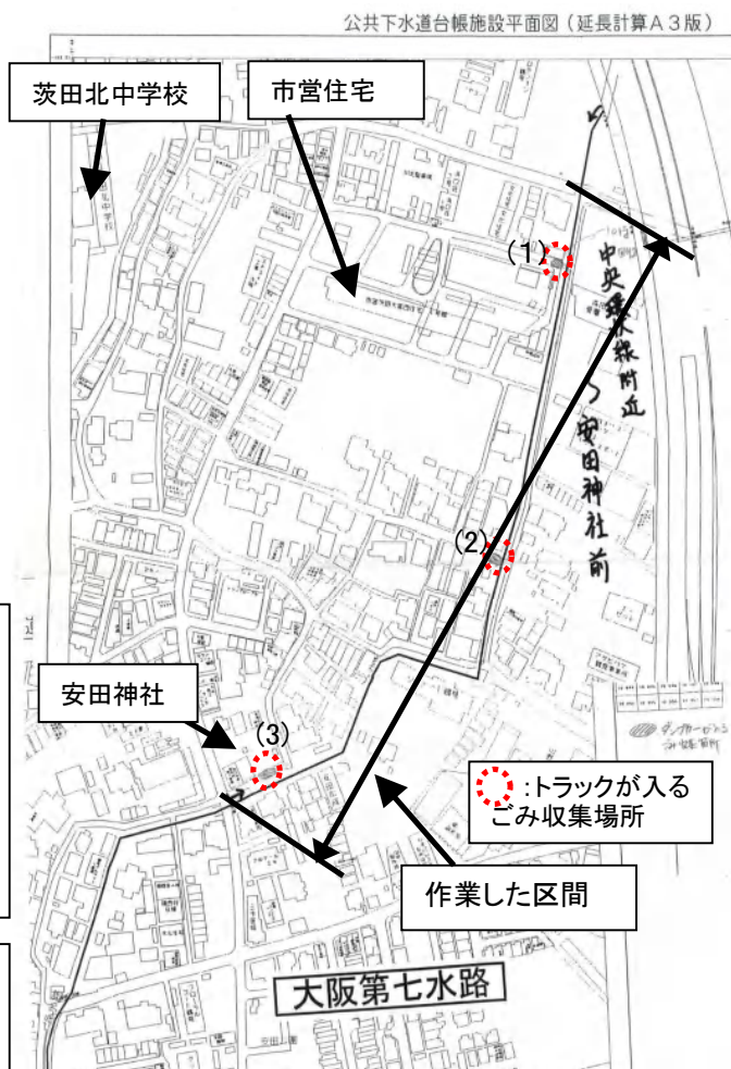
公共下水道台帳施設平面図(延長計算A3版)
