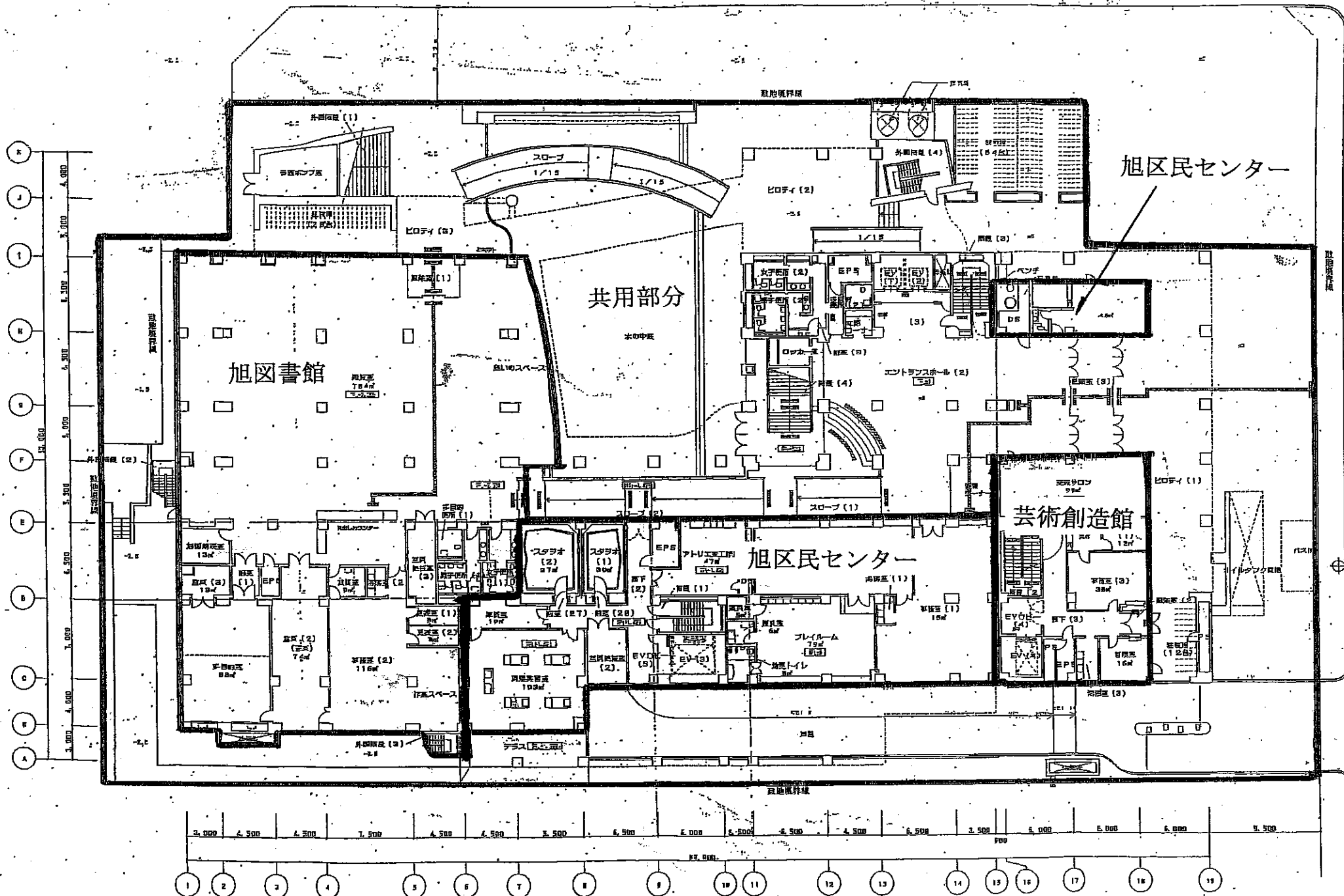
1階平面図
