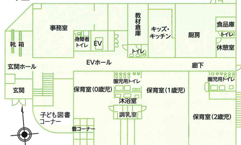
なにわのもり保育園 平面図
