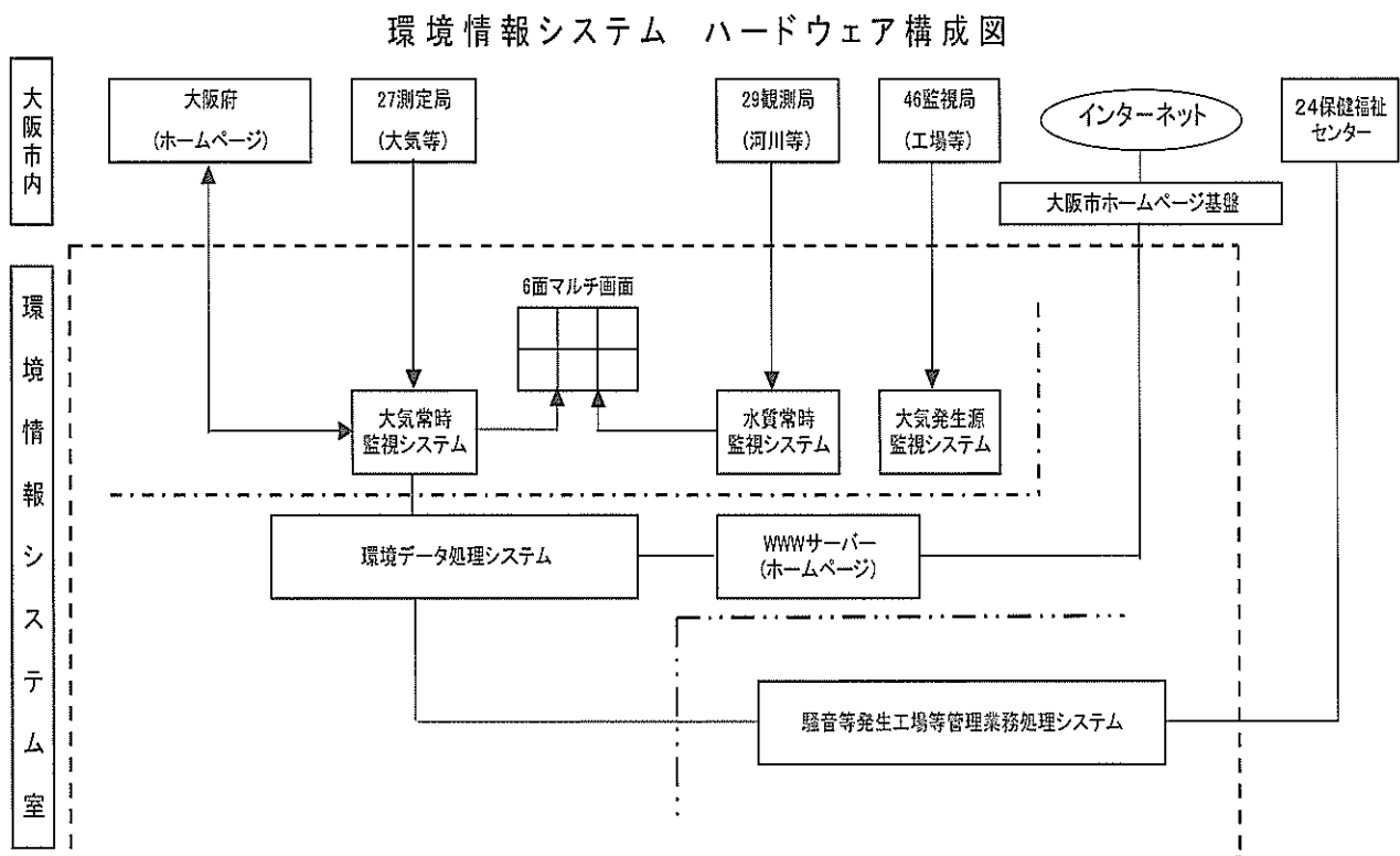
図1-7-1 環境情報システムのハードウェア構成
