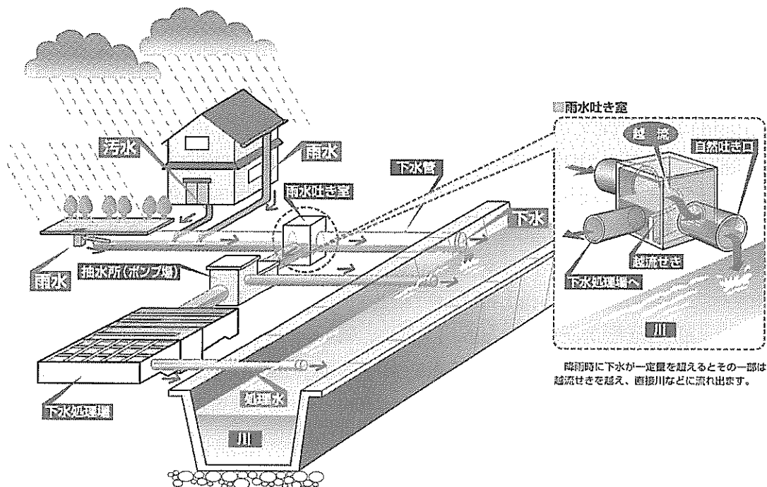
図 1-3-8 合流式下水道の現状
