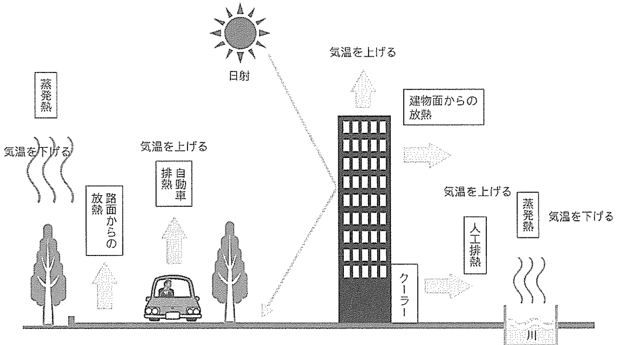
図2-1-1 ヒートアイランド現象の仕組み
