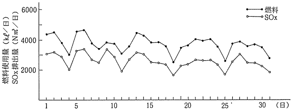
図1-16 燃料使用量およびSOx排出量の経日変化 (59年3月)
