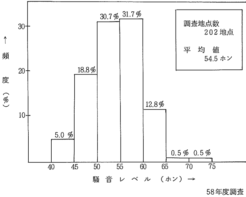
図3-18 地域騒音の騒音レベル別頻度（昼間）
