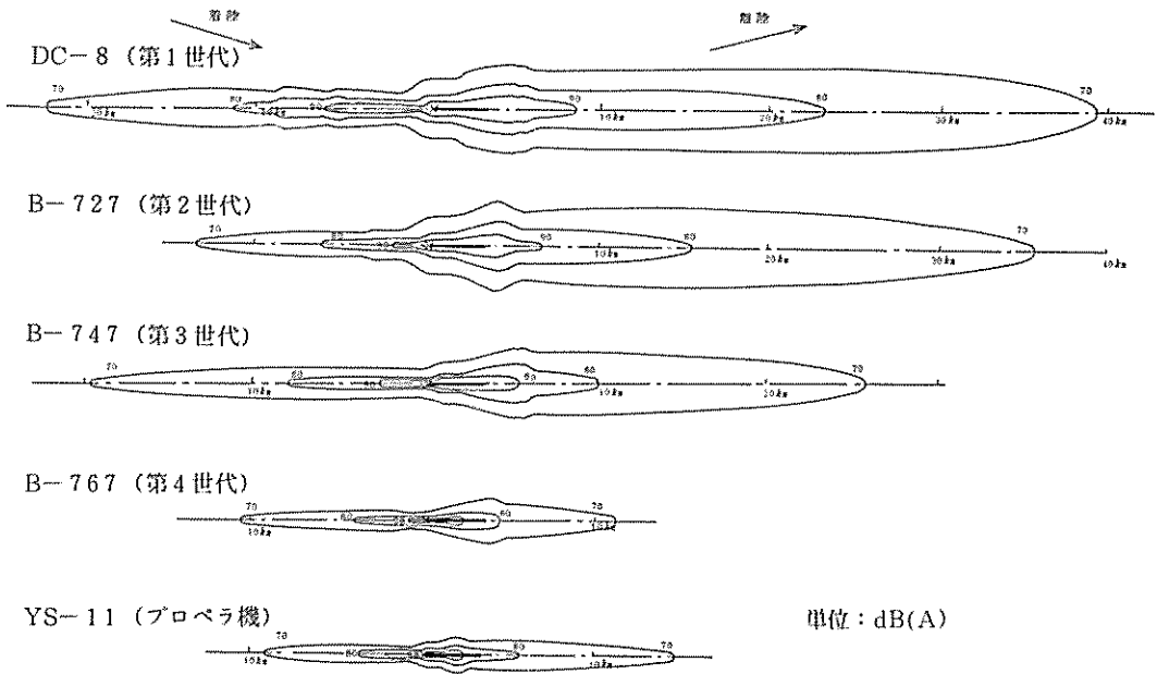
図3-17 機種別騒音コンターの比較
