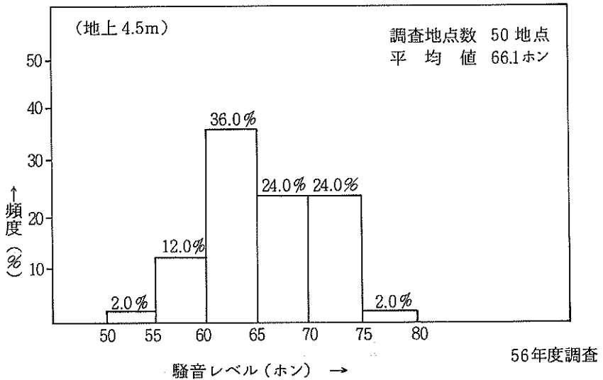
図3-16 高速道路における騒音レベル別頻度 (昼間)
