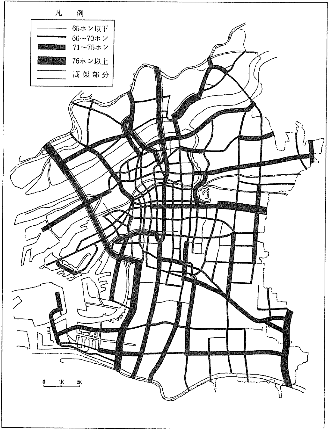
図3-15 幹線道路の路線別騒音レベル(昼間)
