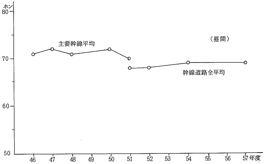
図3-14 幹線道路における自動車騒音の経年変化
