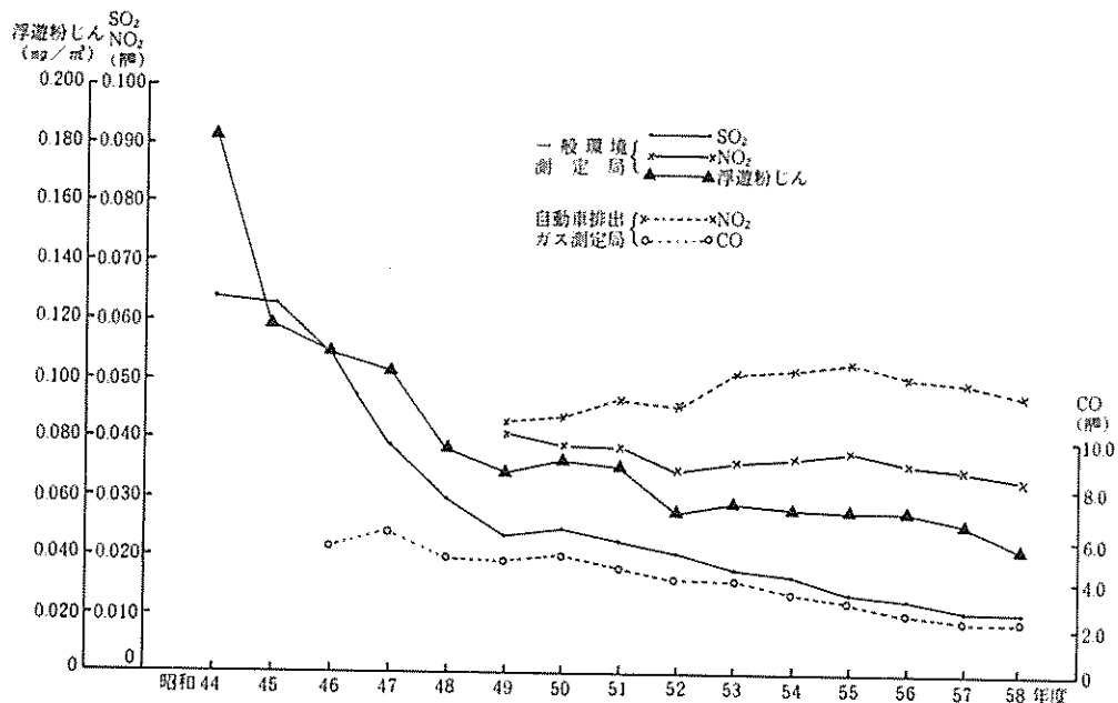
図1-5 主な大気汚染物質の市内平均濃度の経年変化
