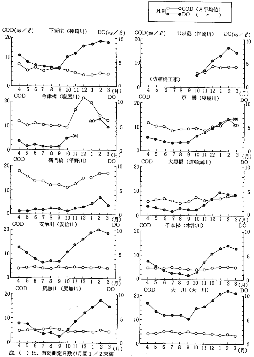
図 2-10 河川観測局による測定結果の月別変化 (58年度)
