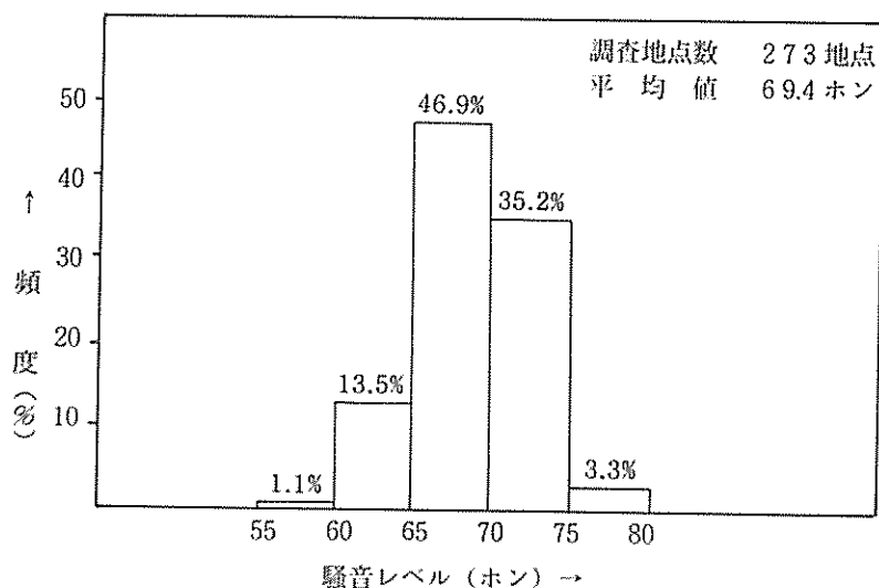
図3-13 幹線道路における騒音レベル別頻度（昼間）
