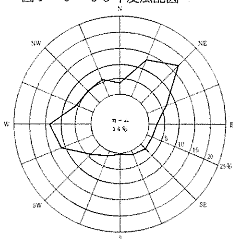
図1-6 58年度風配図
