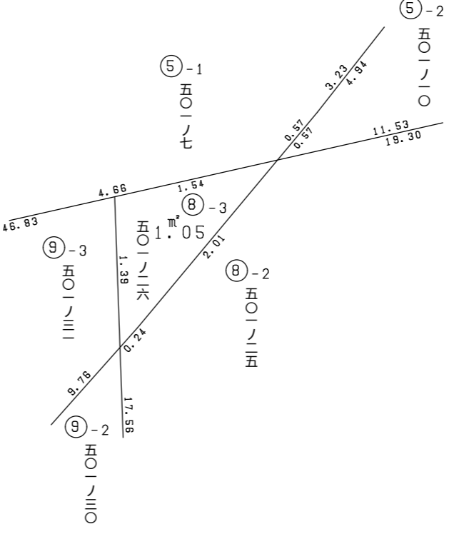
拡大図 縮尺 1 : 50
