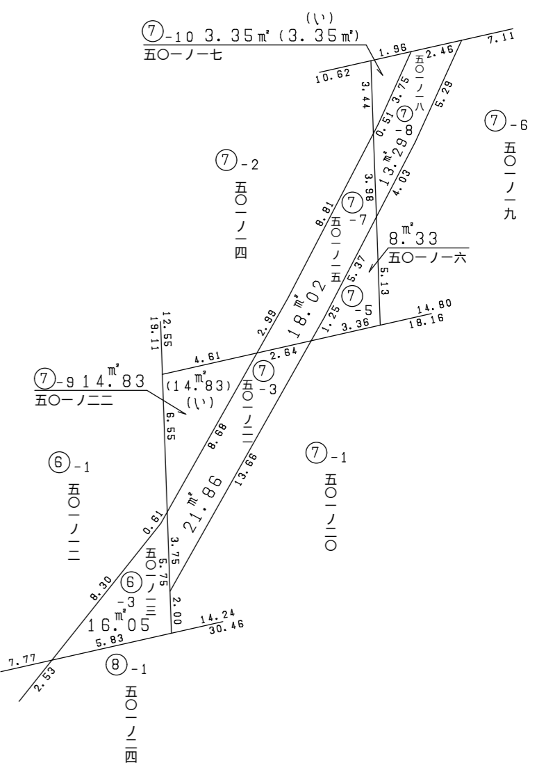
拡大図 縮尺 1 : 250
