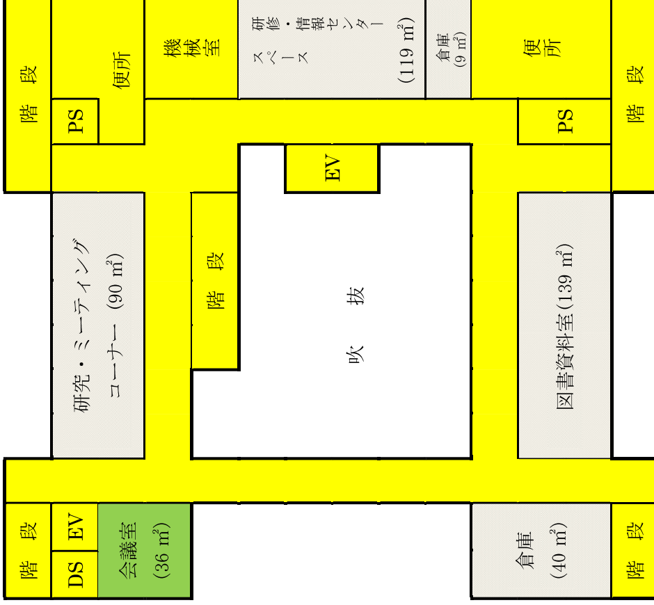
2階平面図
