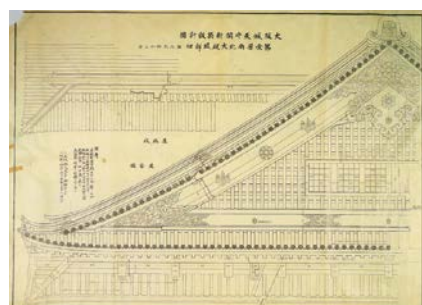
大阪市指定文化財 昭和6年復興大阪城天守閣設計原図等関係資料のうち 第一層南北大破風詳細
