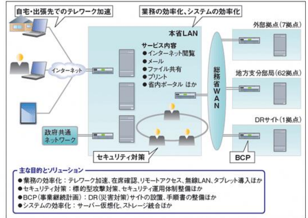
図6 総務省ネットワーク構成図
