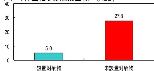
自動火災報知設備設置状況と建物火災1件当たりの焼損面積 (H22)
