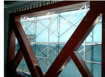
鉄骨ブレースによる耐震化
