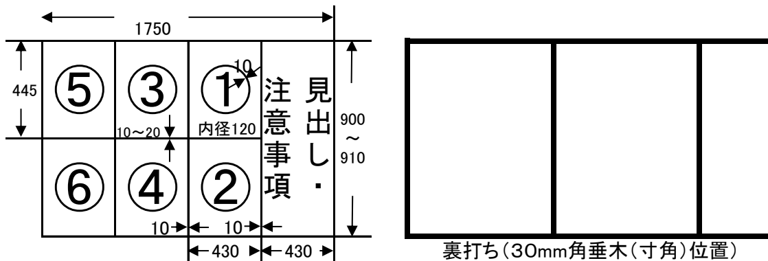
大阪市議会議員〇〇区選挙区補欠選挙ポスター掲示場の様式(単位:mm)
