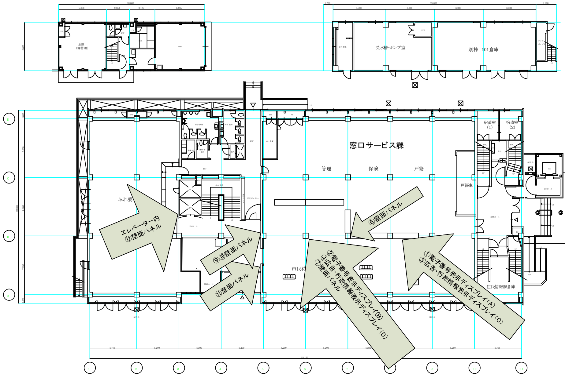
1階 平面図
