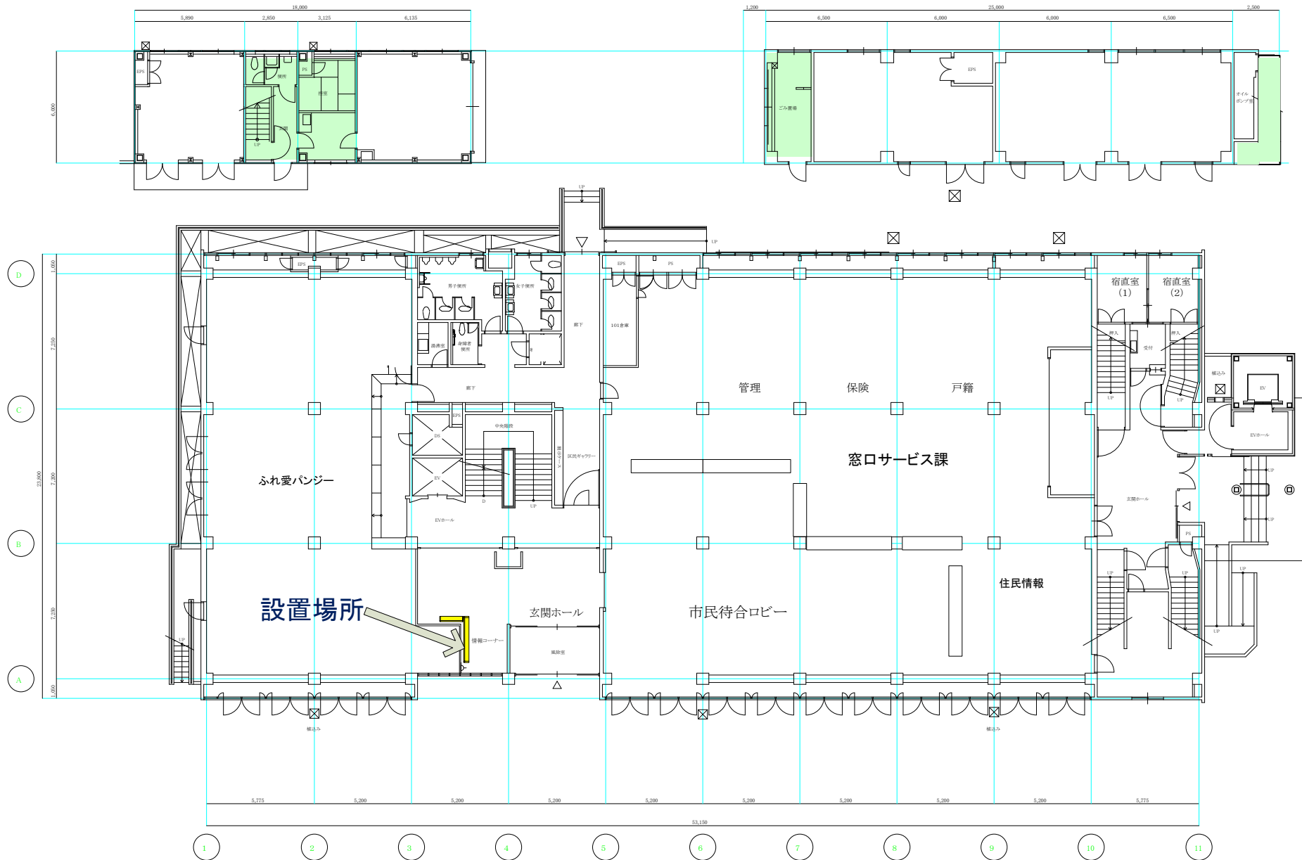
1階 平面図
