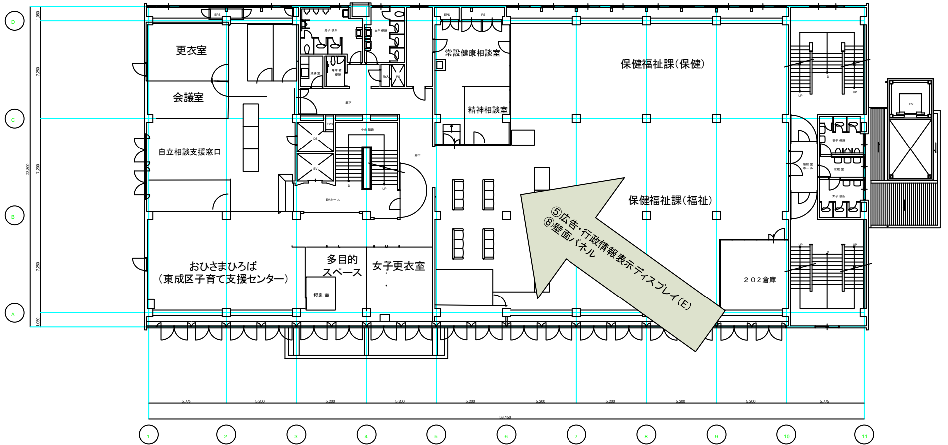
2階 平面図
