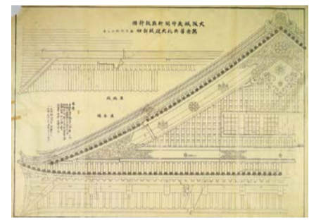
大阪府指定文化財 昭和6年復興大阪城天守閣設計原図等関係資料のうち第一層南北大破風詳細
