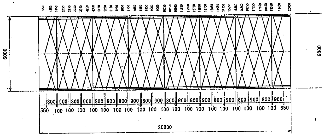
厓根伏圖
