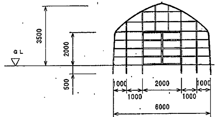
立面図
