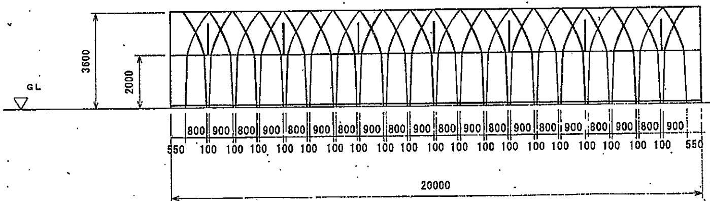
側立面図
