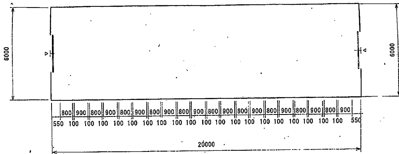
平面図
