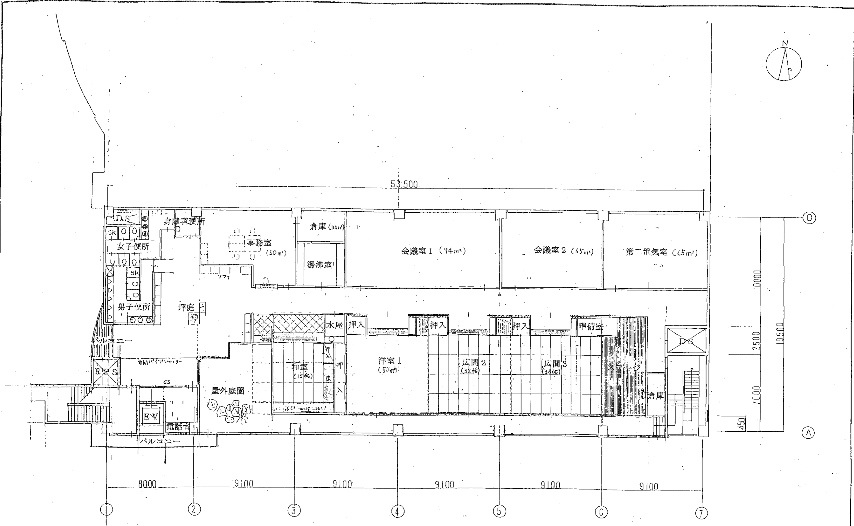
4階平面図 1:200
