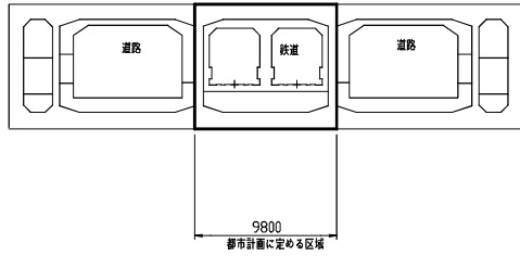
夢咲トンネル部（渡海部） 断面①
