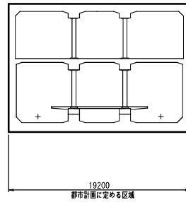
夢洲～車庫線部（線路縦断部） 断面⑥
