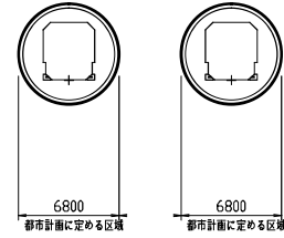
夢洲駅部 断面④
