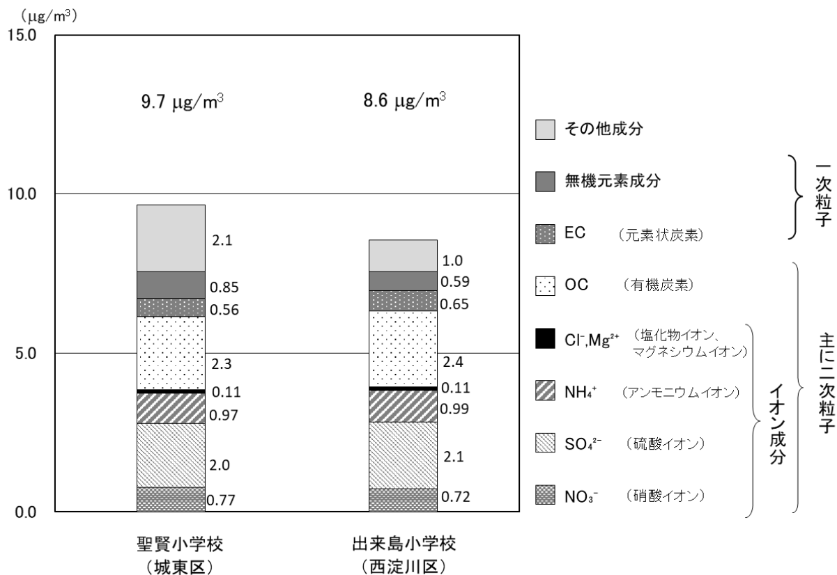
図3-3 微小粒子状物質の令和5年度における成分分析結果（年平均濃度）
