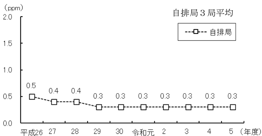
図5-2 一酸化炭素の年平均濃度の推移
