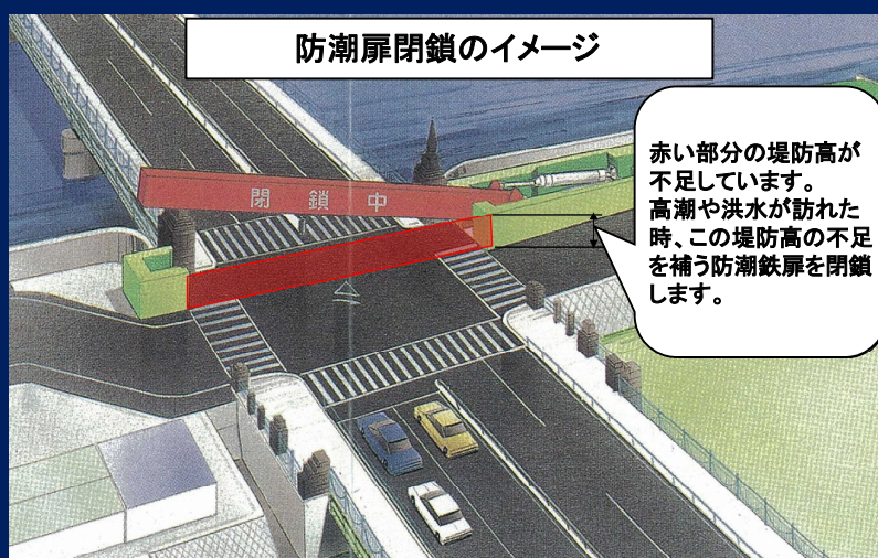
国道2号淀川大橋左岸側 閉鎖のイメージ図
