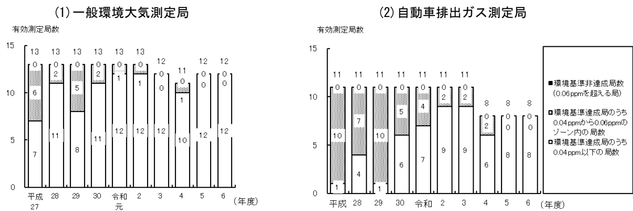
図1-1 二酸化窒素の年平均濃度の推移
