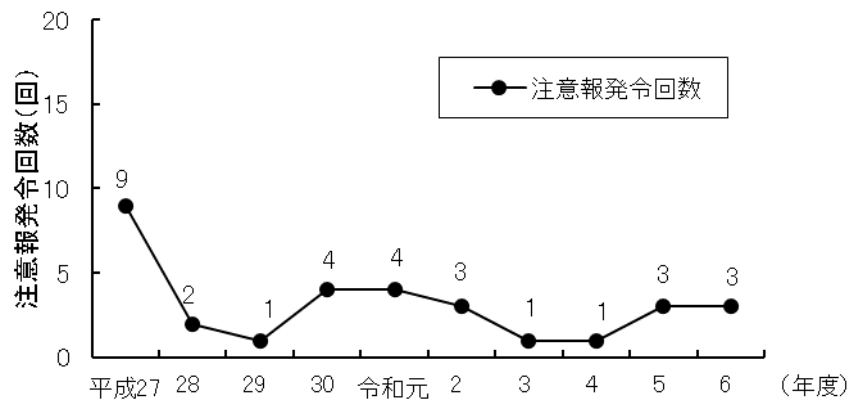
図4-2 光化学スモッグ注意報の発令回数の推移
