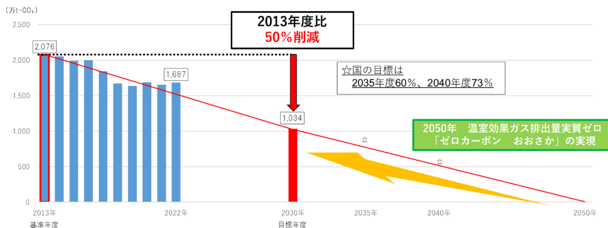
図 2030 年度と 2050 年における削減目標
