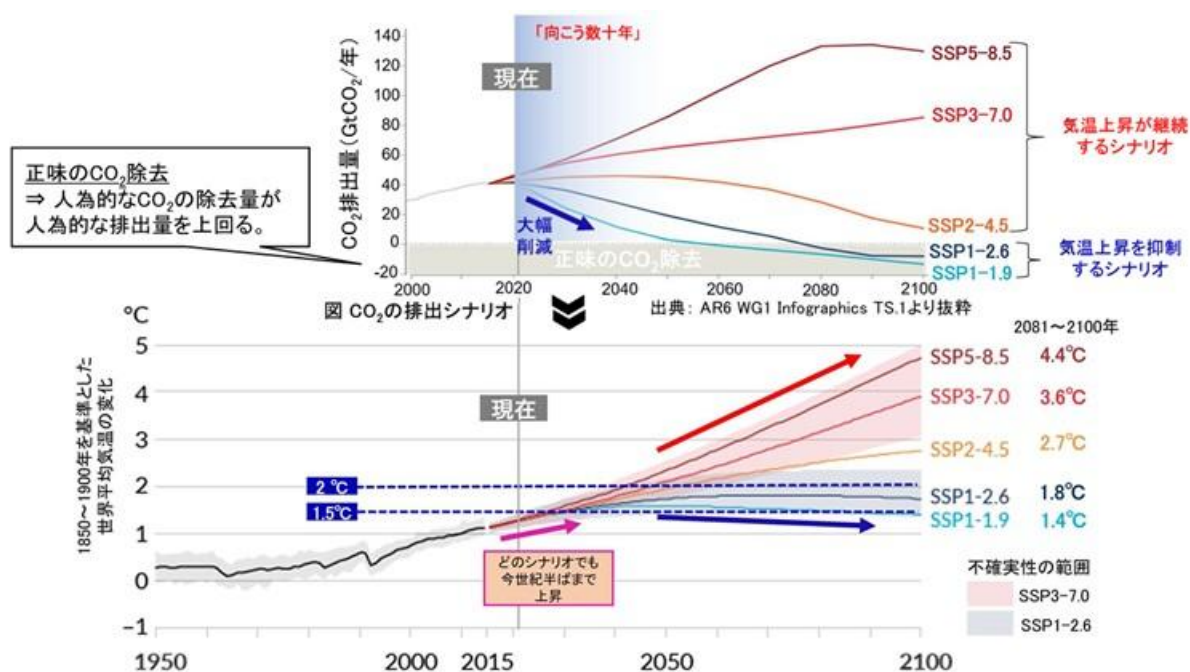
図 CO 2 排出シナリオと 1850～1900 年を基準とした世界平均気温の変化
