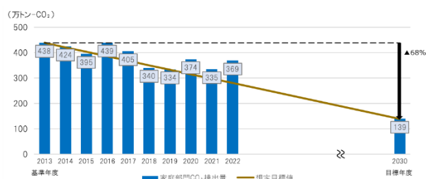
図 家庭部門におけるCO 2 排出量削減の進捗状況
