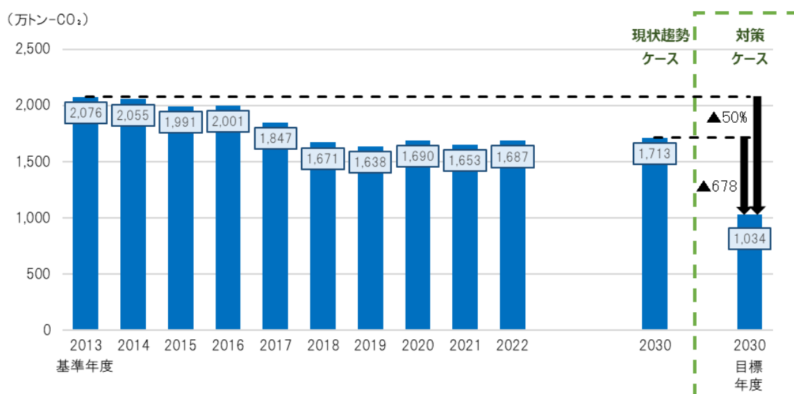
図 大阪市域の温室効果ガス排出量(対策ケース)の推計結果
