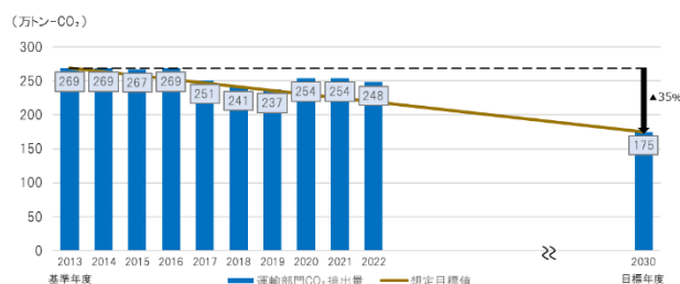
図 運輸部門における CO 2 排出量削減の進捗状況
