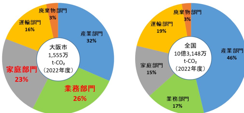
図 CO 2 の部門別排出状況(2022 年度)
