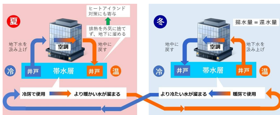
帯水層蓄熱利用のイメージ
