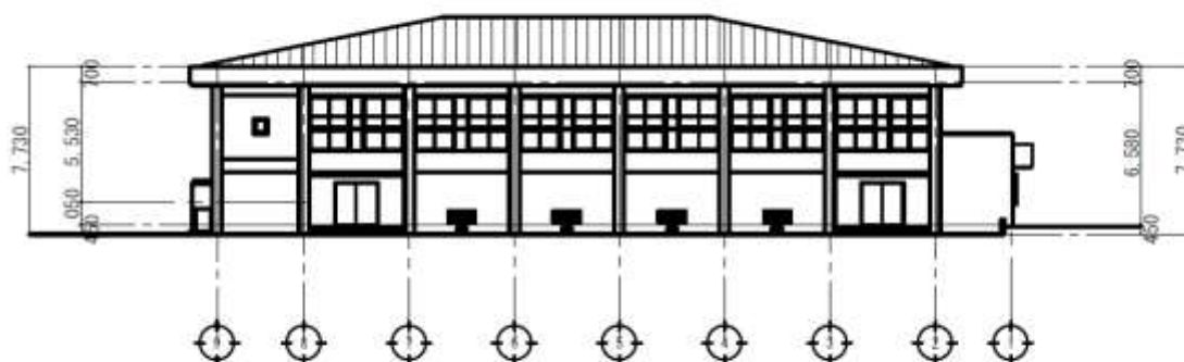
南立面図 1 : 300
