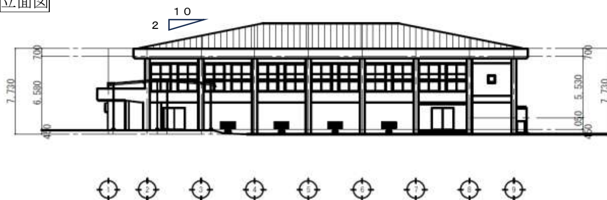
立面図
