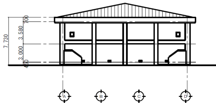
西立面図 1 : 300
