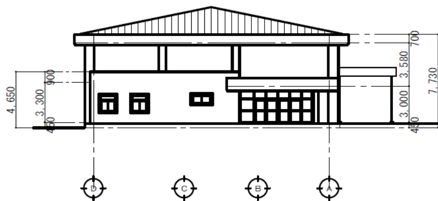
東立面図 1 : 300
