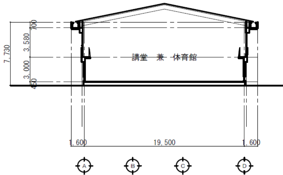
A-A' 断面 1 : 300
