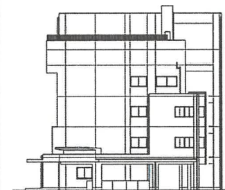
北側立面図
