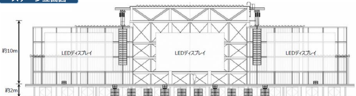
ステージ立面図
