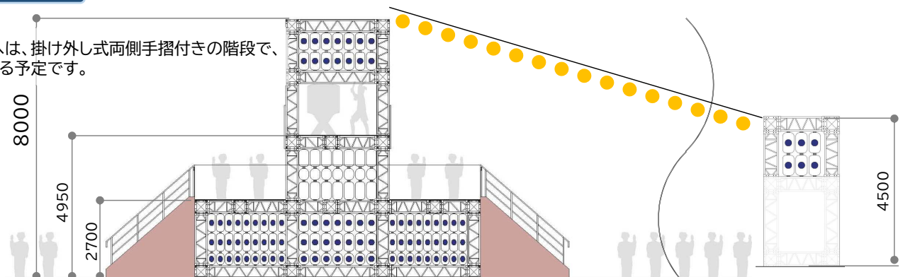
特設檜 立面図
