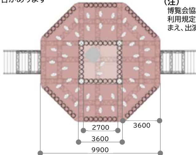
特設檜 平面図
