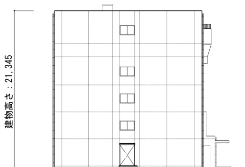
南側立面図
