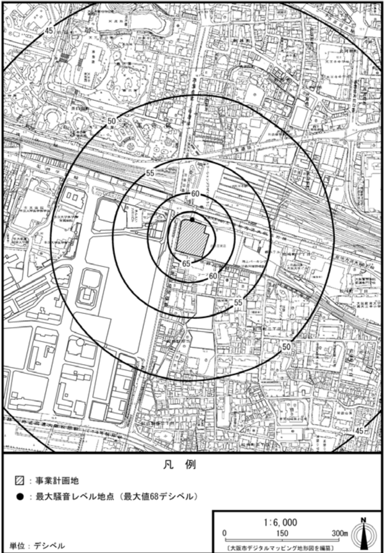
図 5.3.12 建設作業騒音の予測結果(解体工事 2~4 ヶ月目 昼間)
