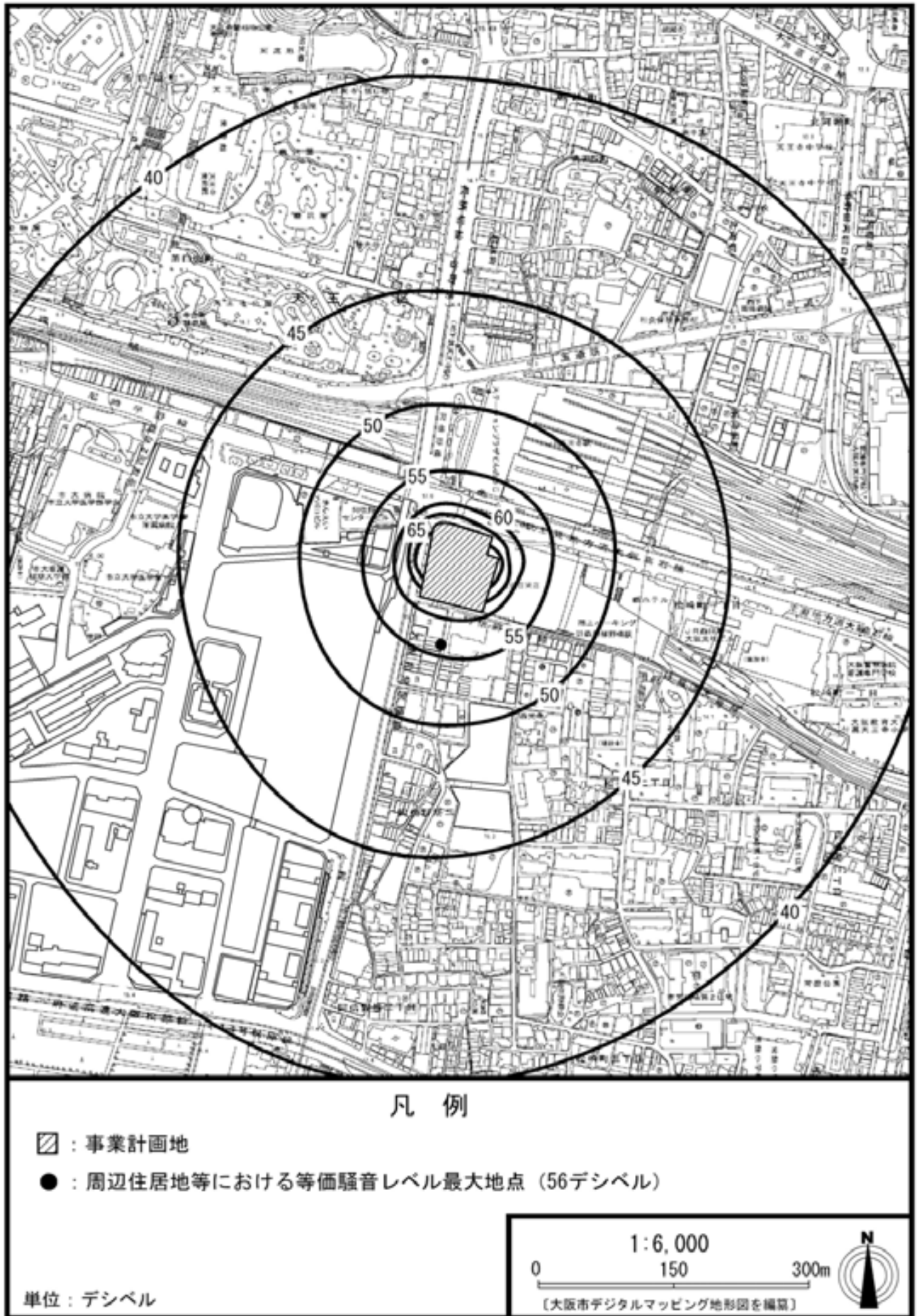
図 5.3.14 建設作業騒音の予測結果(新築工事(掘削工事) 27~40 ヶ月目 夜間)
