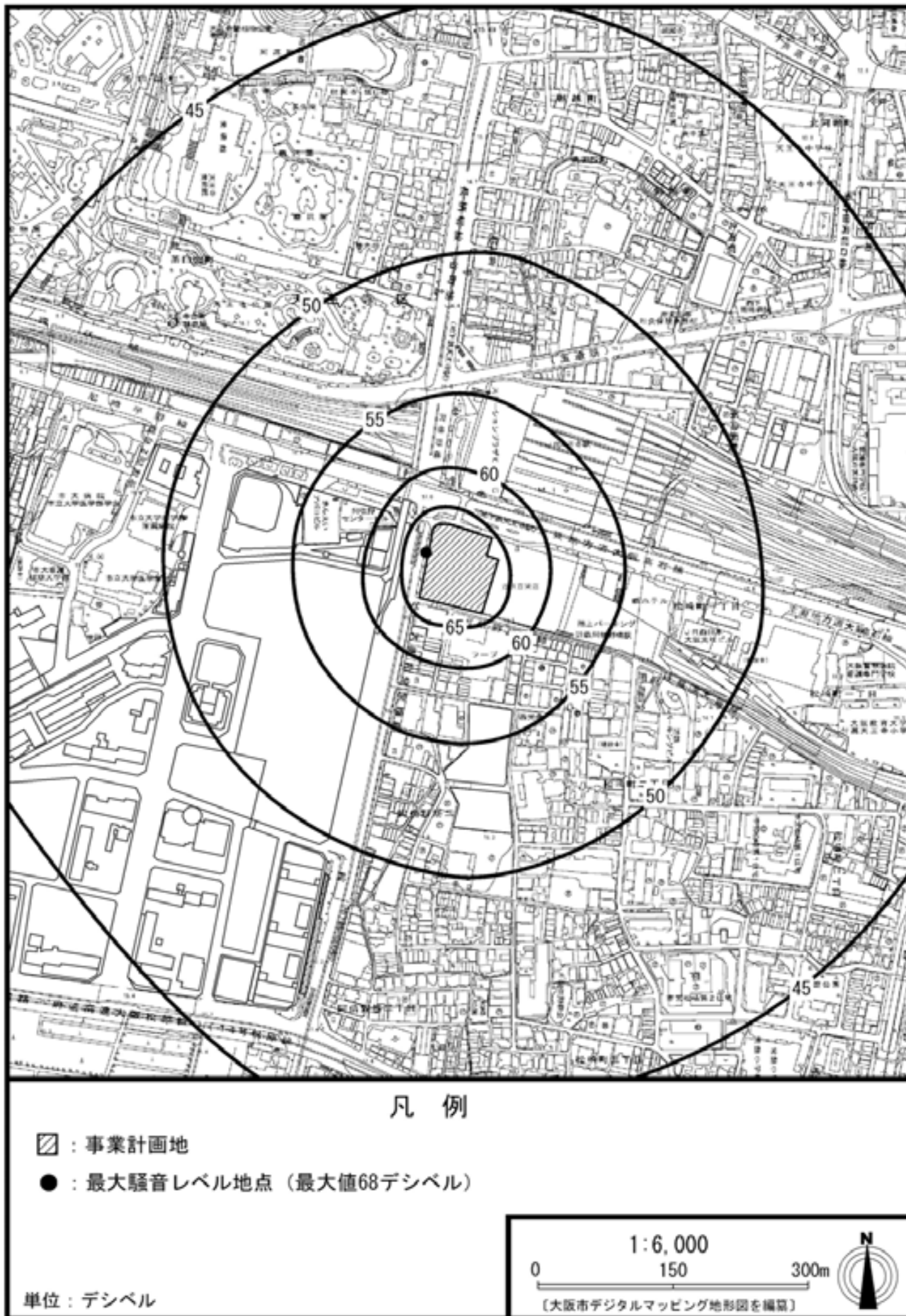
図 5.3.13 建設作業騒音の予測結果(新築工事 13~15 ヶ月目 昼間)
