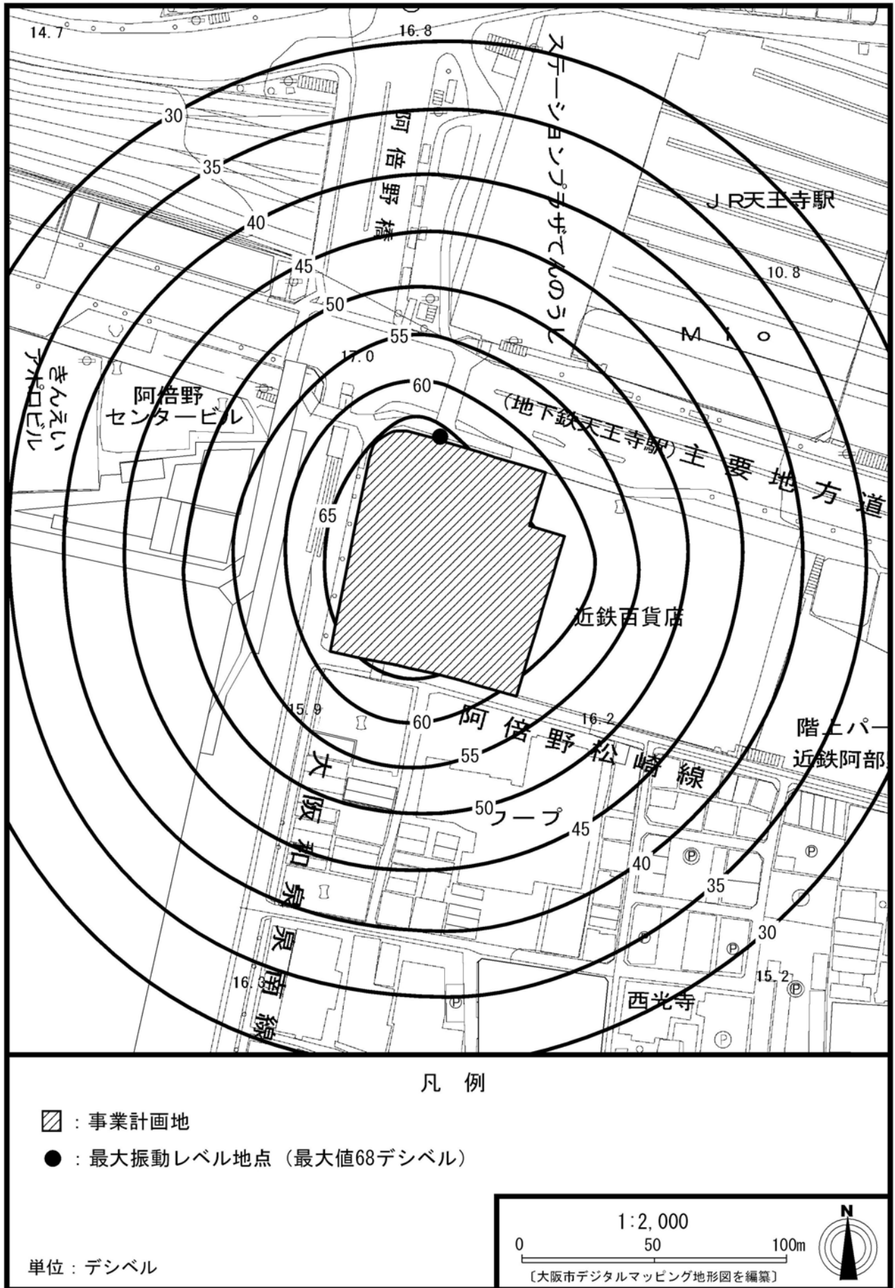
図 5.4.6 建設作業振動の予測結果(解体工事 2~4 ヶ月目 昼間)
