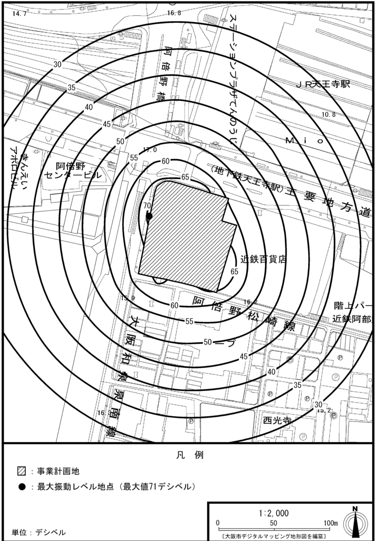
図 5.4.7 建設作業振動の予測結果(新築工事 13~15 ヶ月目 昼間)
