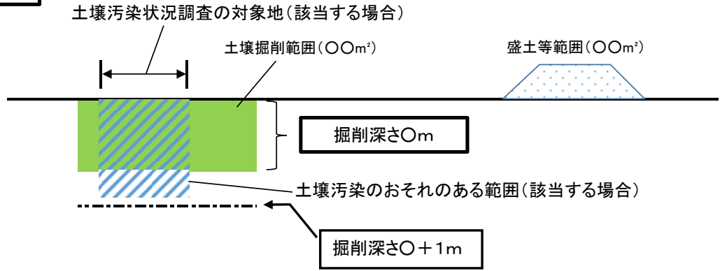
立面図①
