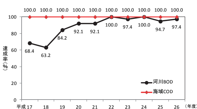
河川のBOD及び海域のCODの環境基準達成率の推移
