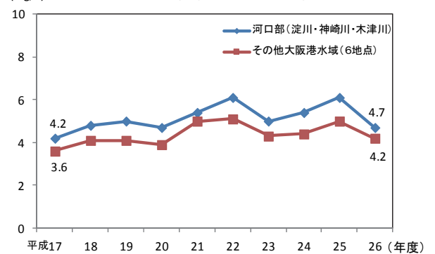
大阪港のCOD(表層年平均値)の推移
