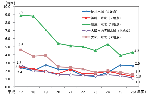
市内河川の水域別のBOD(年平均値)の推移
