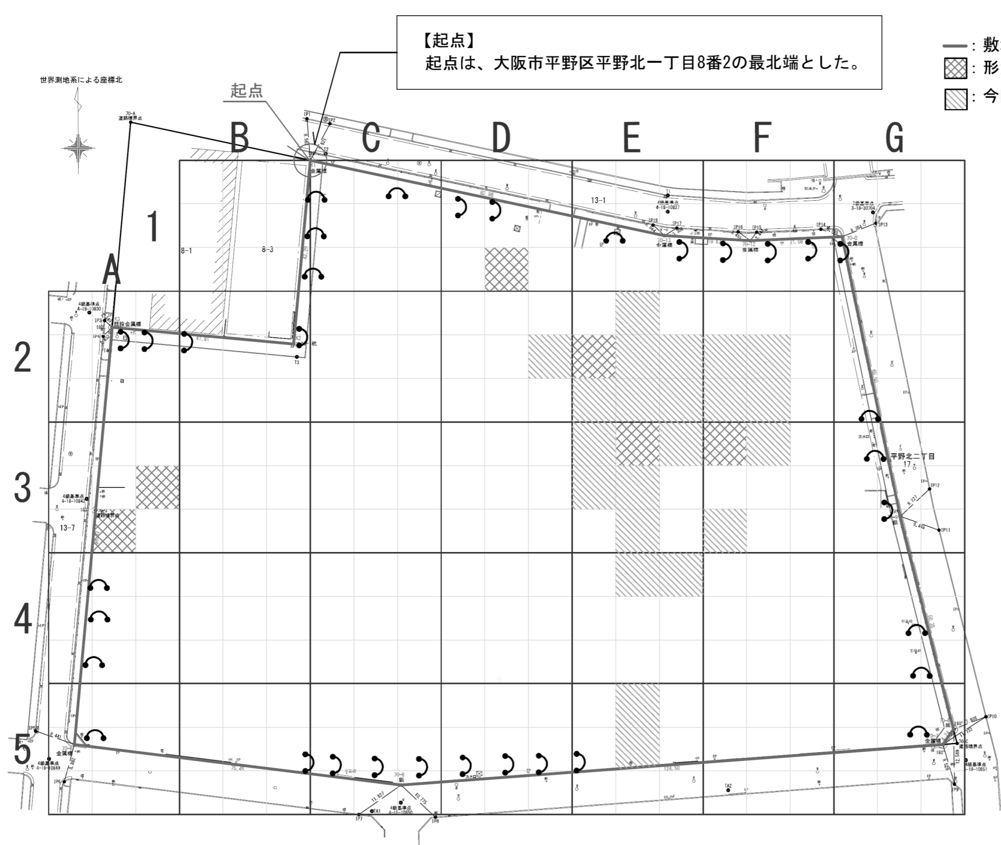
形質変更時要用届出区域図
