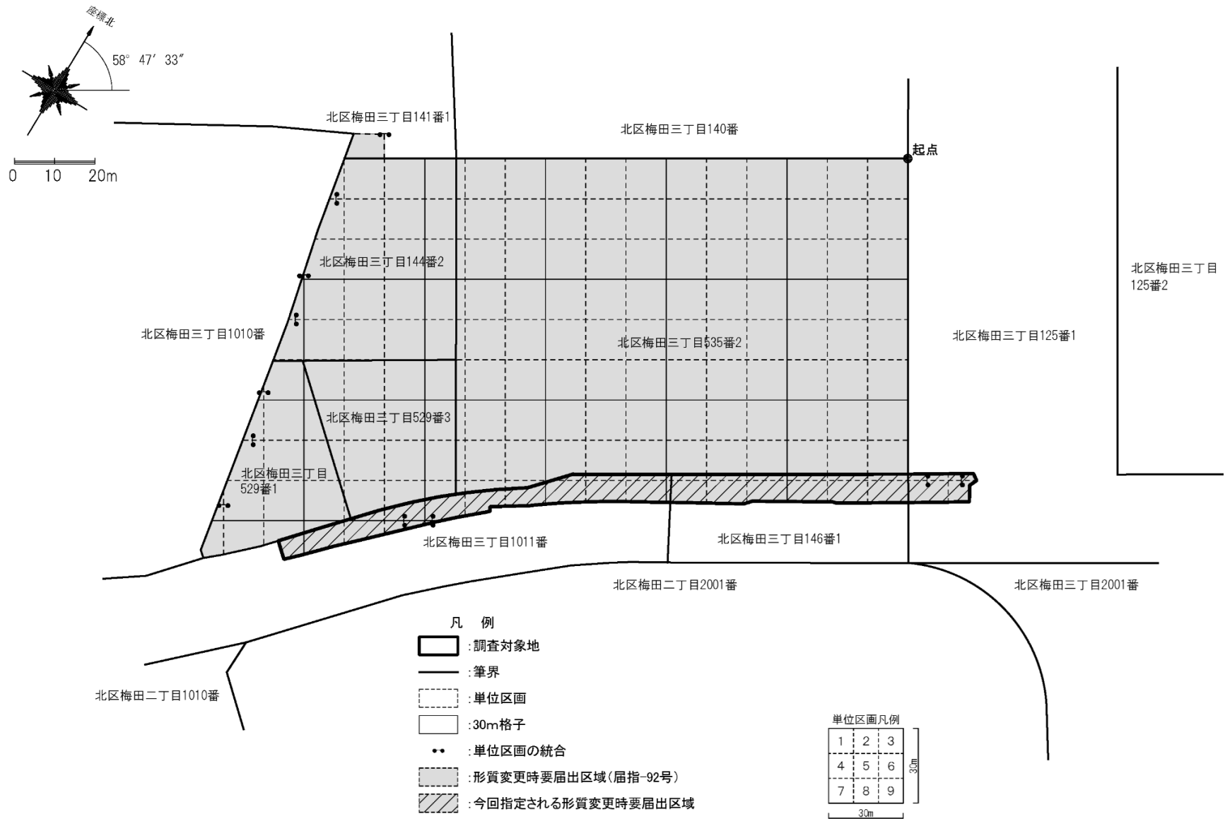
形質変更時要届出区域図面
