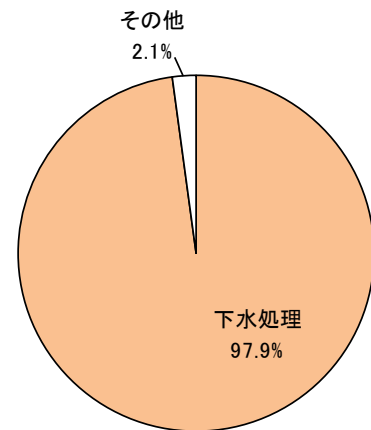
図 2 - 3 \text{CH}_4 排出状況
