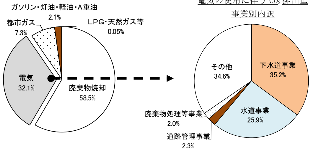
図2-2 CO 2 排出状況 ※四捨五入の関係で数値の合計が 100 にならない場合がある。
