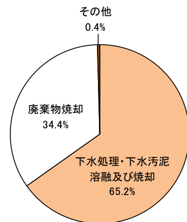
図 2 - 4 \text{N}_2\text{O} 排出状況
