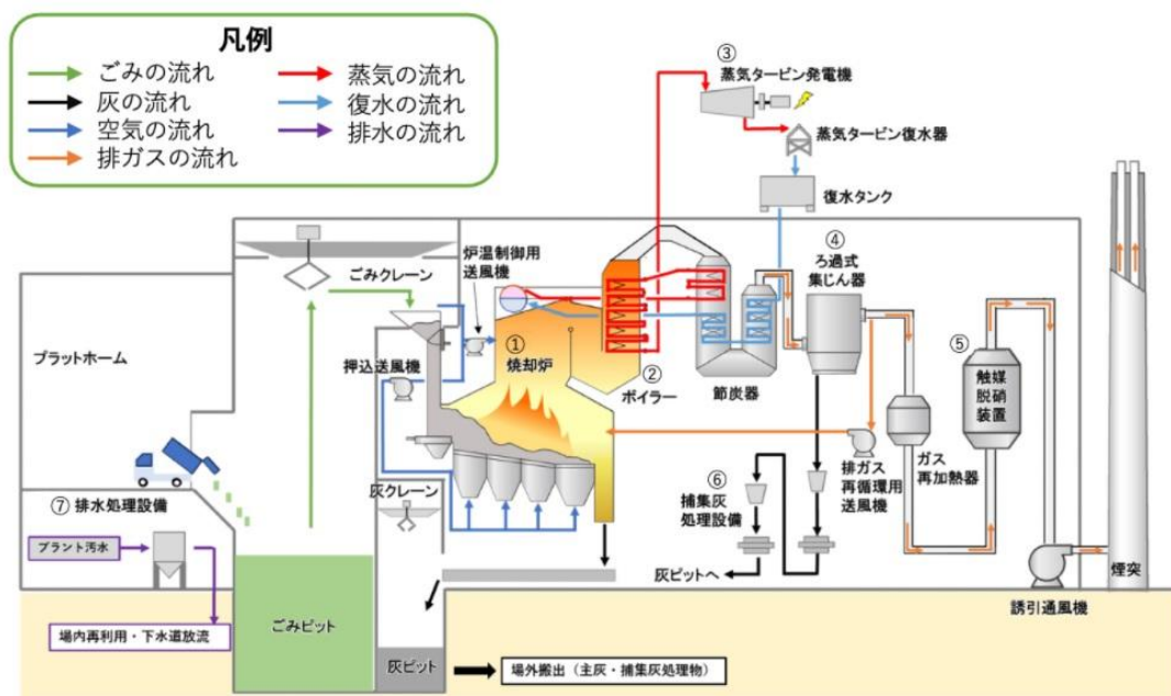
鶴見工場の熱回収フロー図
