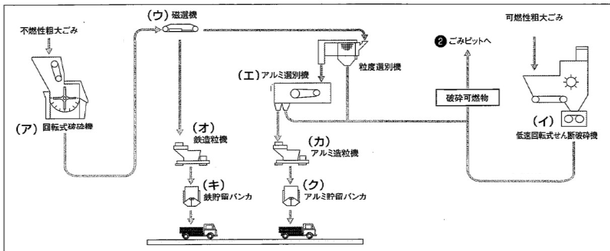
粗大ごみ破碎設備のフローシート（例：舞洲工場）
