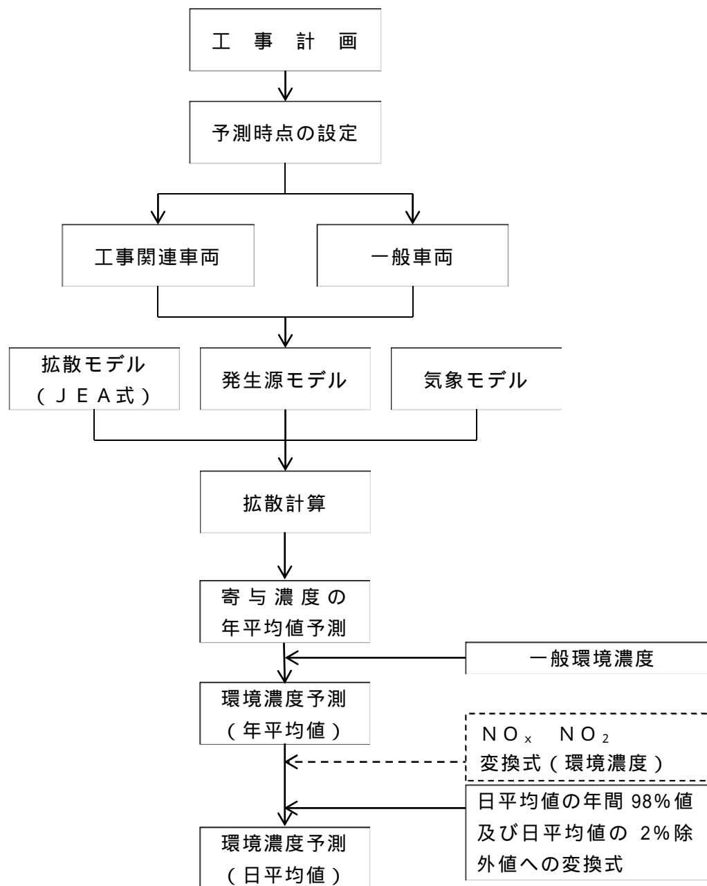
図 5-2-18 工事関連車両の走行により発生する排出ガスの予測手順
