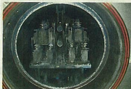
真空加熱分離装置でのコンデンサ処理(引渡性能試験) (左：処理前、右：処理後)
