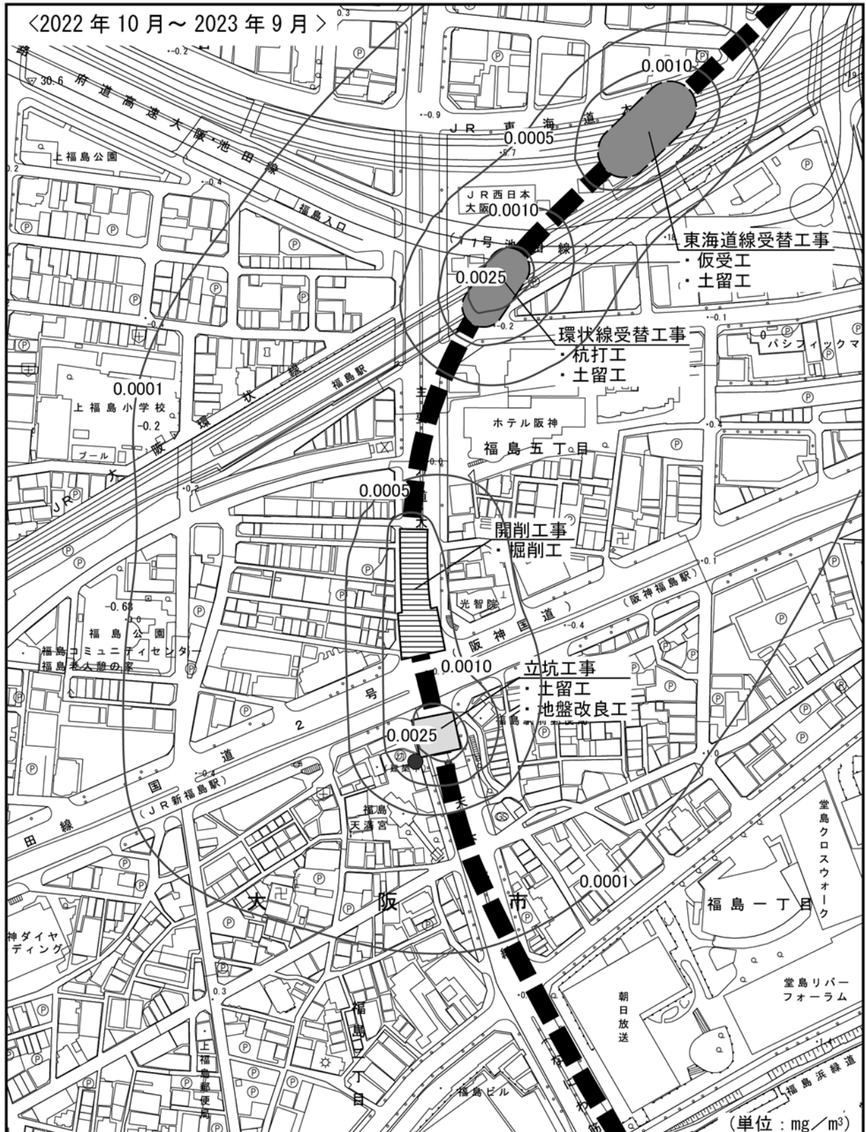
図6.2.11(2) 建設機械による寄与濃度 （浮遊粒子状物質、1.5m高さ） 【国道2号開削部】
