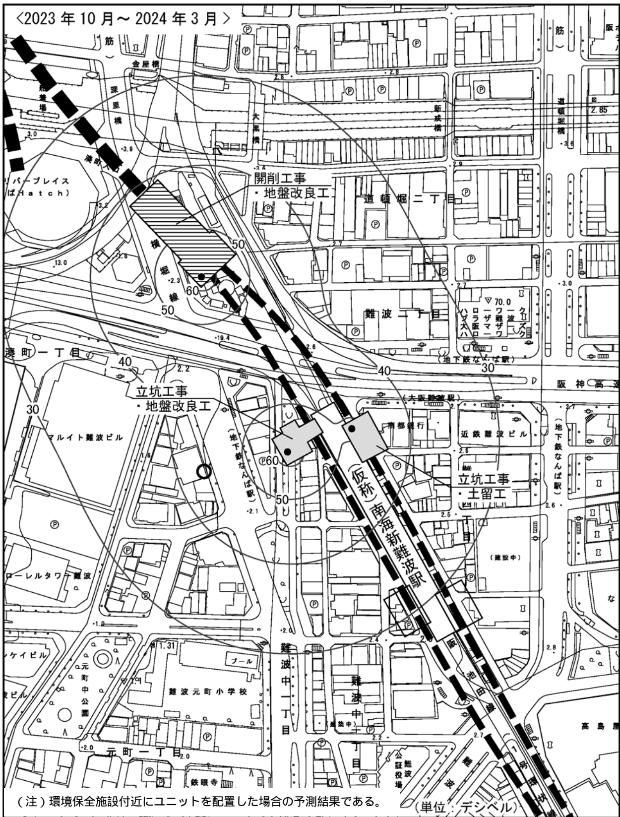
N 1:3,000 0 50 100m 図6.6.9(6) 建設機械による振動 (振動レベルの80%レンジ上端値、地盤上) 【南海新難波駅立坑】
