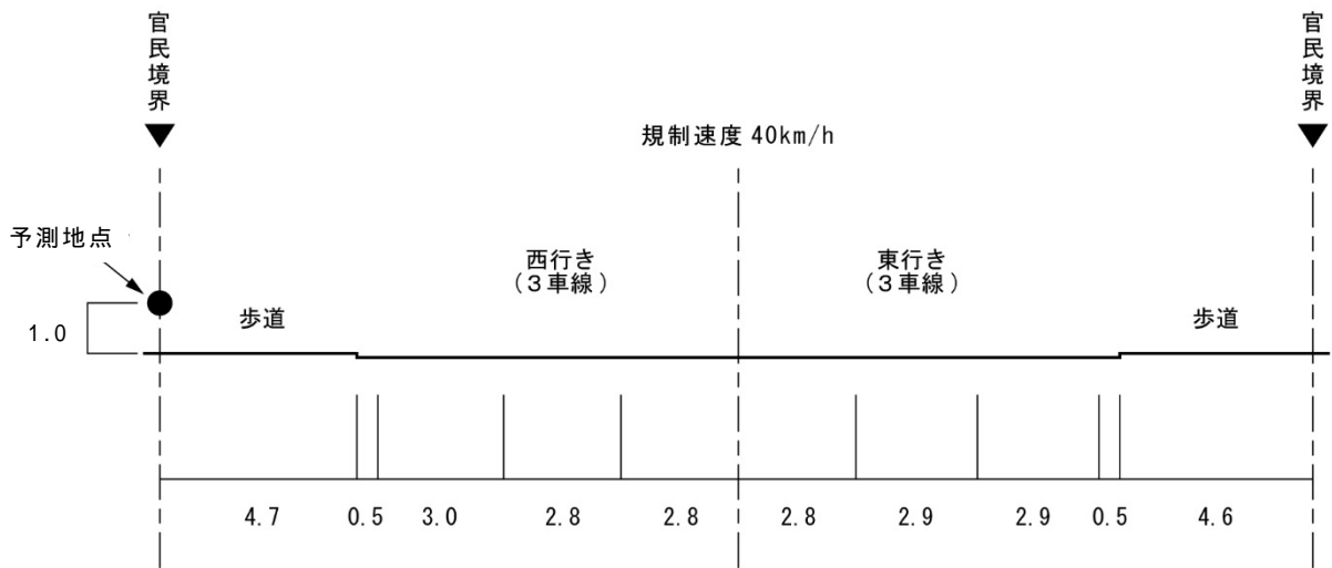
図 5-2-13(2) 交通 2 における道路断面
