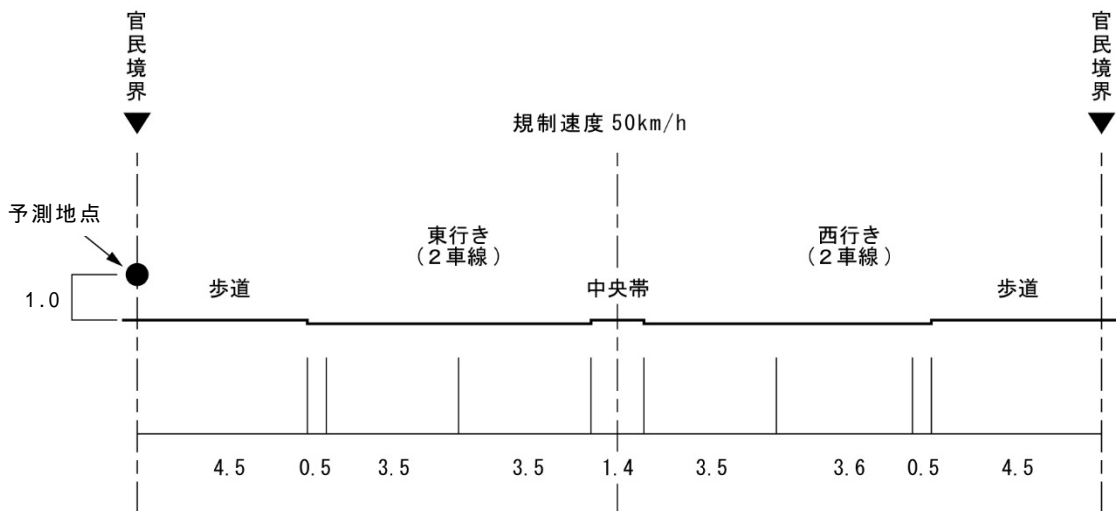
図 5-2-13(3) 交通 3 における道路断面
