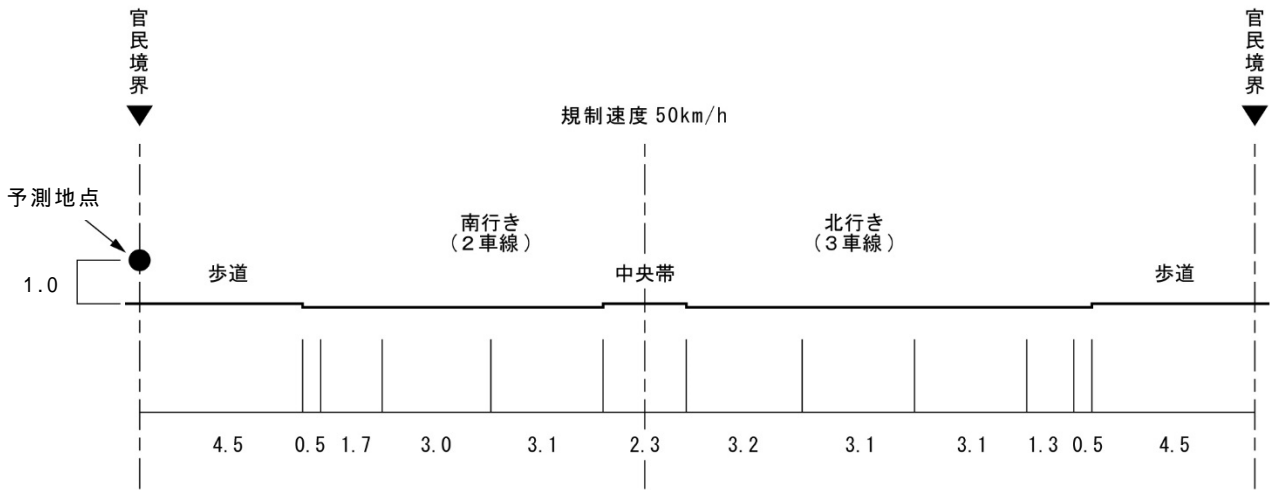
図 5-2-13(1) 交通 1 における道路断面
