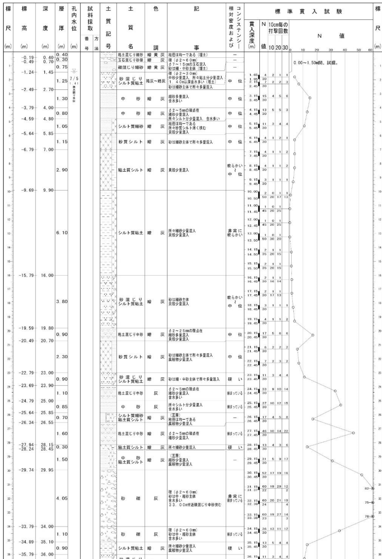
図 5-7-4(1) 土質柱状図 (北 2 地点) 次頁に続く
