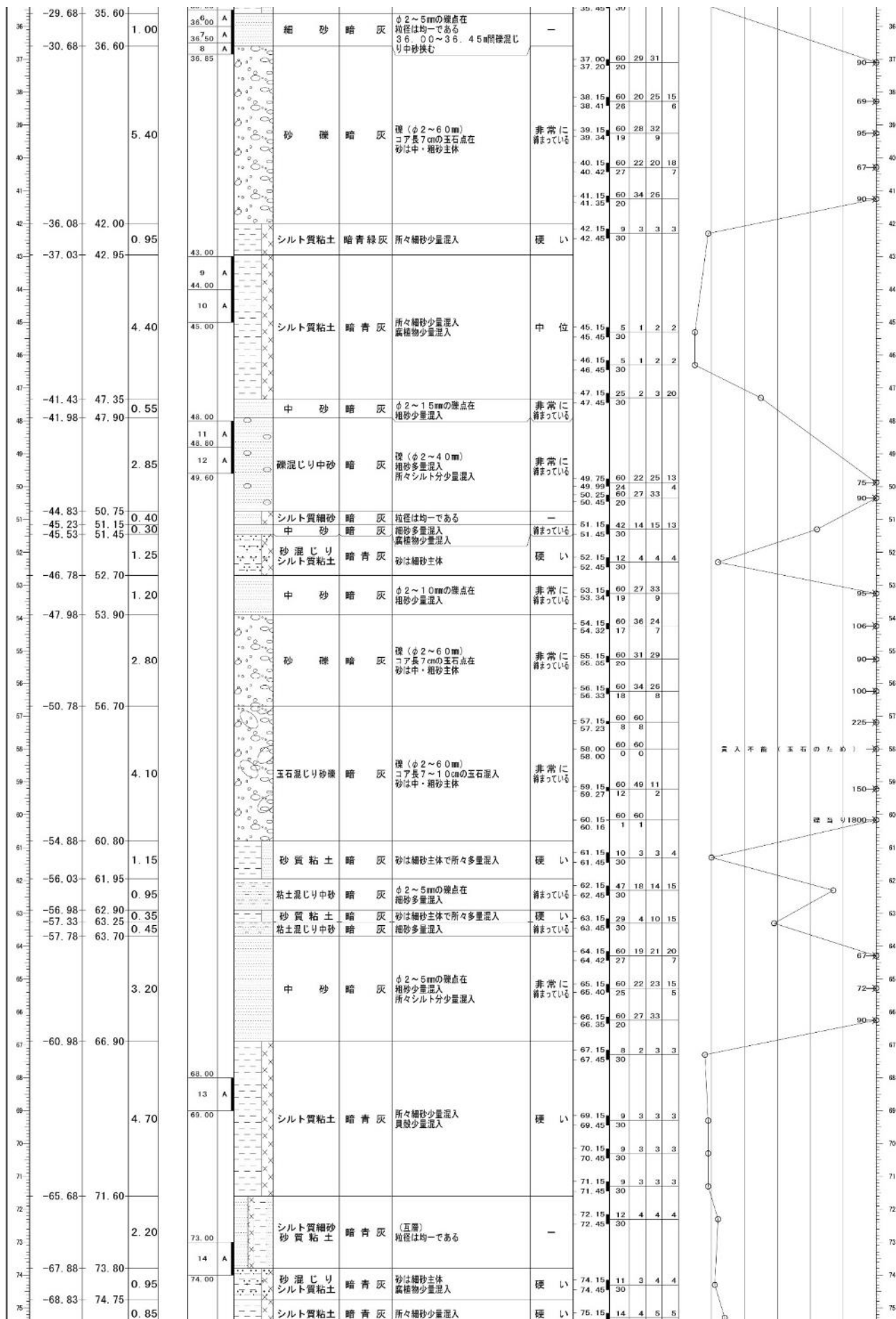
図 5-7-5(2) 土質柱状図 (南1地点) 次頁に続く
