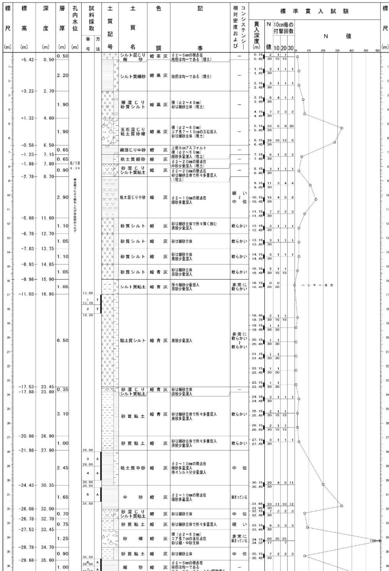
図 5-7-5(1) 土質柱状図 (南 1 地点) 次頁に続く
