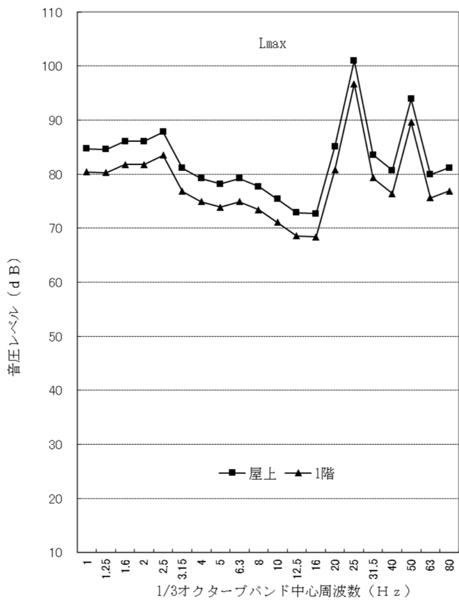
図 6.2.3 周波数別の音圧レベル（最大の地点：No.3）
