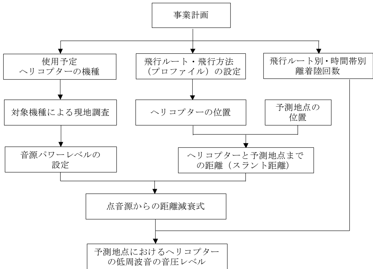
図 6.2.2 ヘリコプターの運航に伴う低周波音の予測手順
