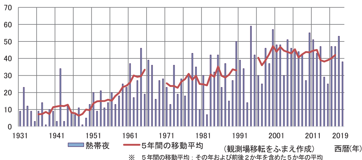
日数(日) 大阪市域における熱帯夜日数の経年変化(1931~2019)
