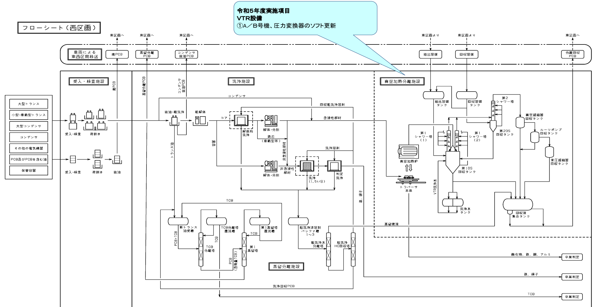
図-1 大阪PCB処理事業所（西棟）「令和5年度実施」の長期保全計画実施箇所（表-2から抜粋）
