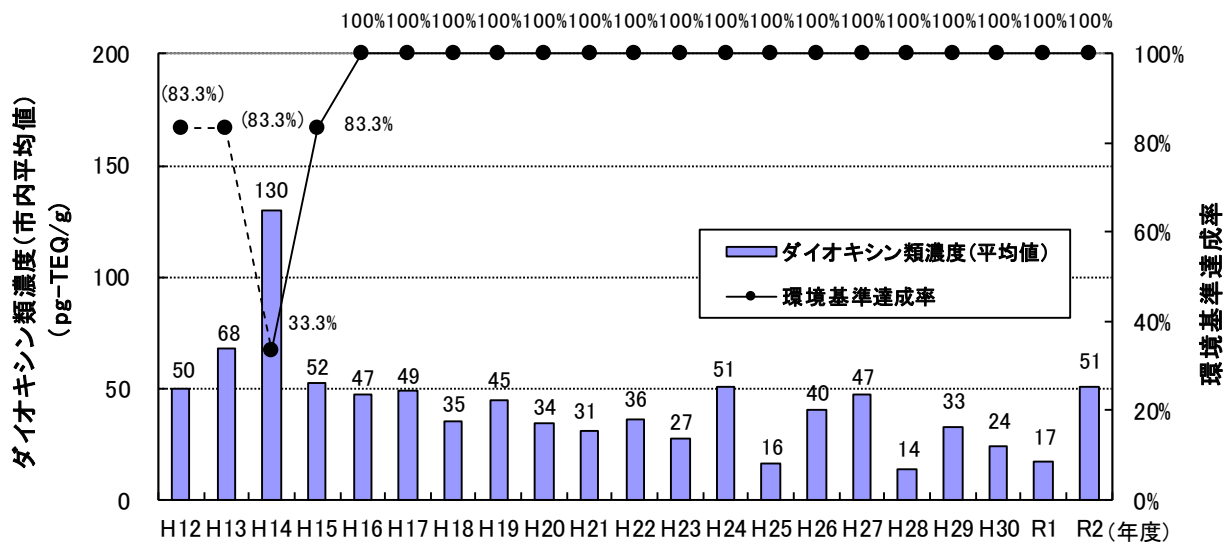
図 7 ダイオキシン類常時監視結果の推移（海域底質）
