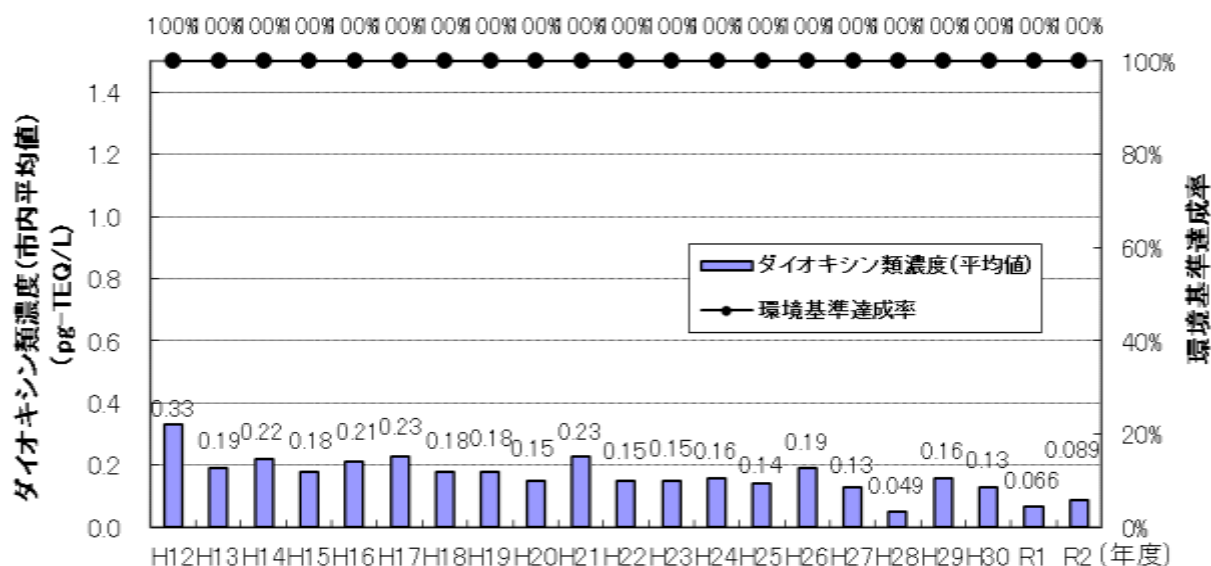
図 4 ダイオキシン類常時監視結果の推移（海域水質）
